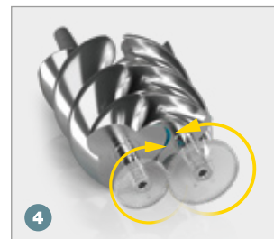
4 Camera della soffiante completamente svuotata
