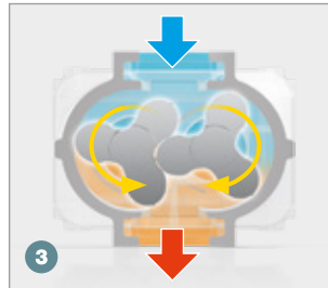
3 Espulsione dell'aria
