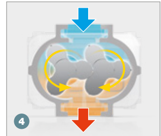
4 Camera della soffiante completamente svuotata
