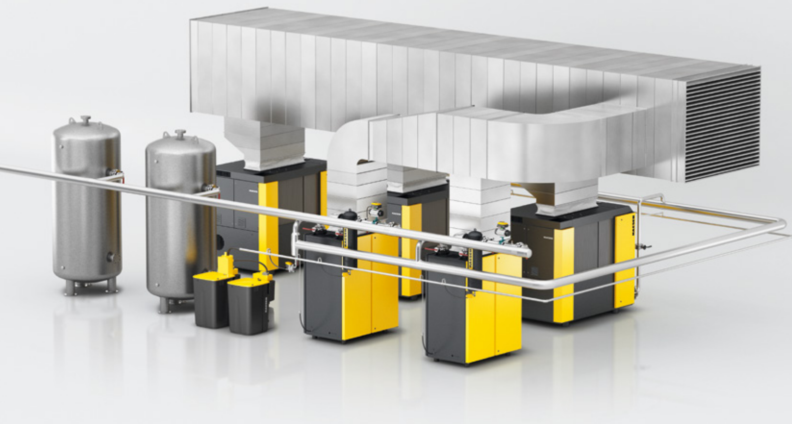
Esempio di stazione con collettore per compressori ed essiccatori a ciclo frigorifero
